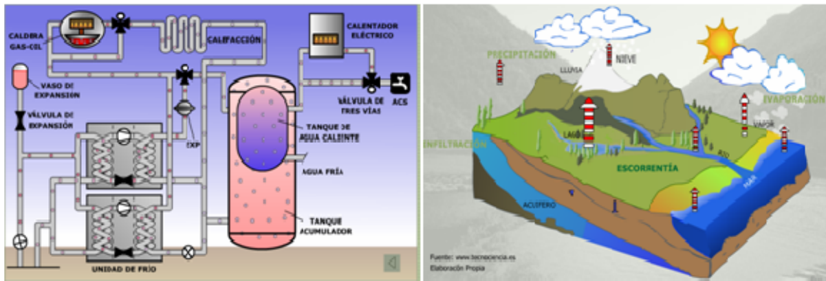
Figura 4. Ejemplos de animaciones en 2D. a) un circuito geotérmico. b) Un esquema del ciclo hidrológico.
