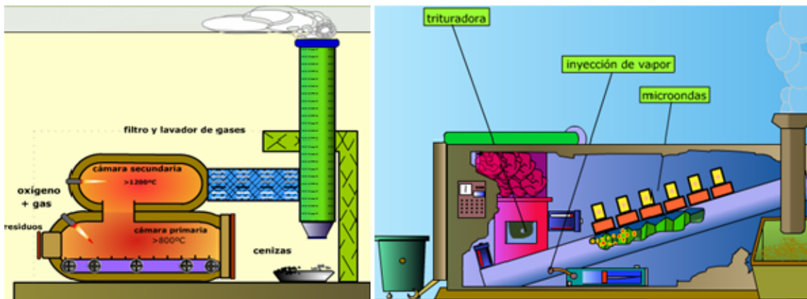
Figura 2. Esquemas simplificados de tratamiento de residuos sanitarios.
