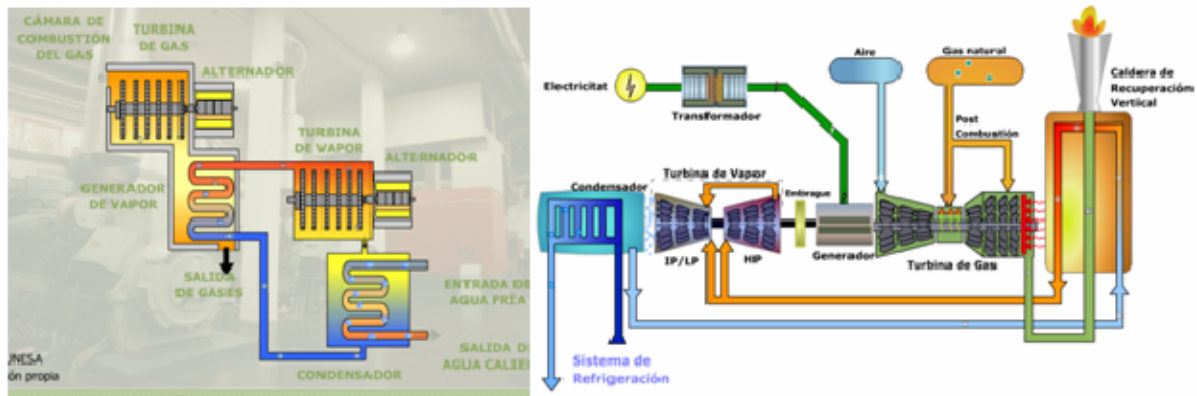
Figura 1. Formas de representar un proceso productivo
