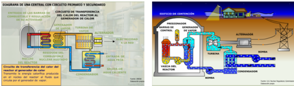
Figura 3. Esquema funcionamiento de una central nuclear y su representación en forma de circuitos.
